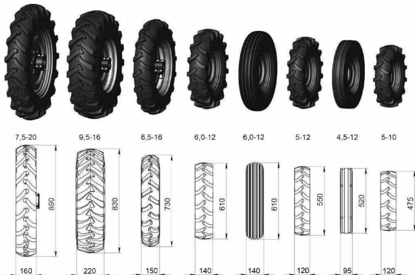
Рис. 15.1. Размеры колес.
