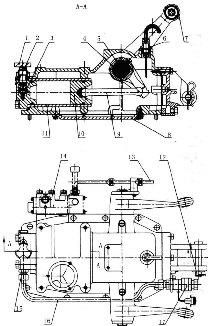
Рис. 18.8. Гидроподъемник трактора ТЕ-254.
