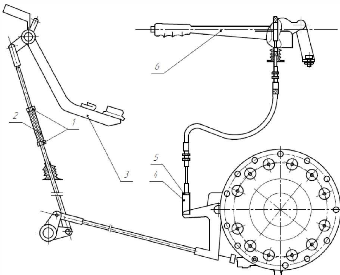
Рис. 17.1. Регулировка управления тормозами.
