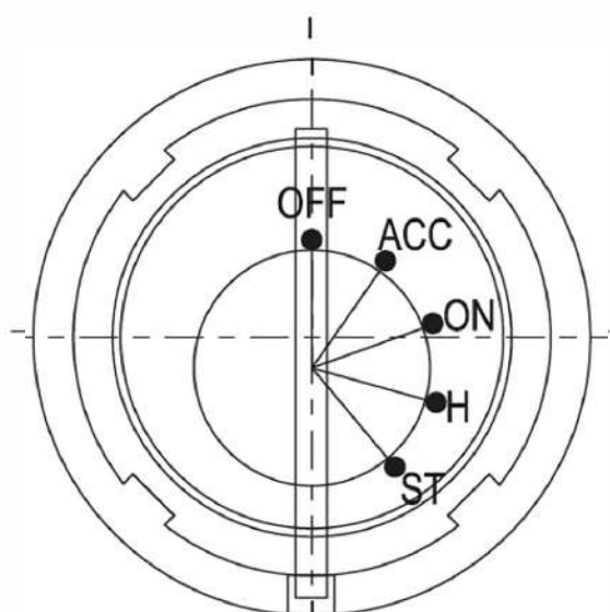
Рис. 9.1. Замок зажигания.
